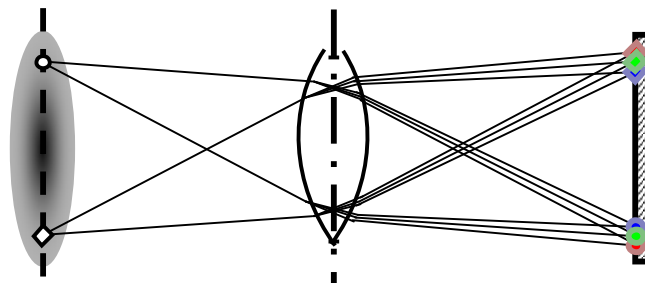
Figura: Aberraciones cromáticas laterales que se producen al pasar la luz por un cristal
