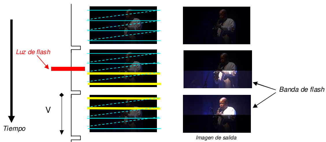
Figura: Explicación del fenómeno de Bandas de Flash en sensores CMOS
